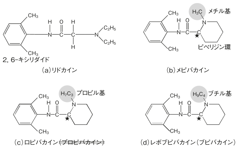
図 1 化学構造式
