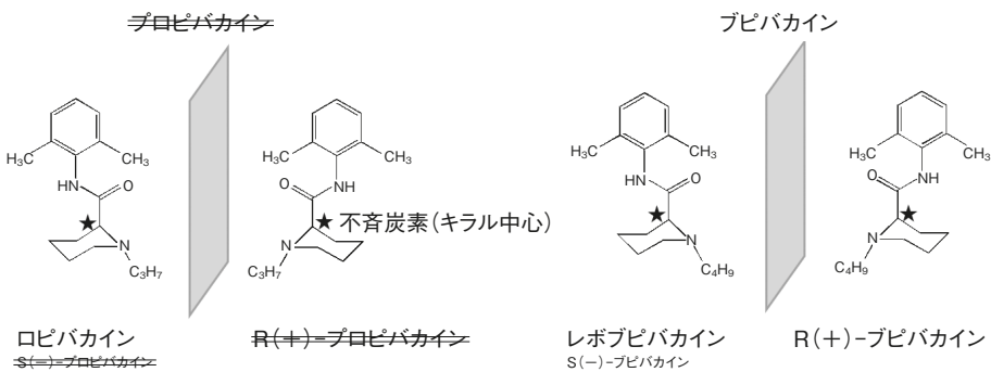
図 2 プロピバカインとブピバカインの鏡像異性体
