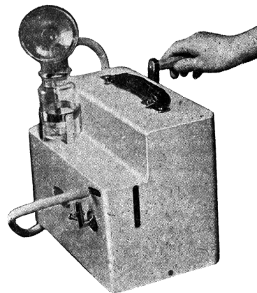
チエム手廻式搾乳器
